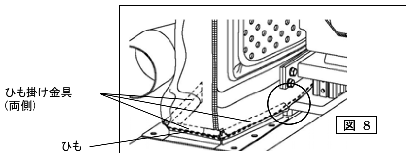
ひも掛け金具付近の詳細図
